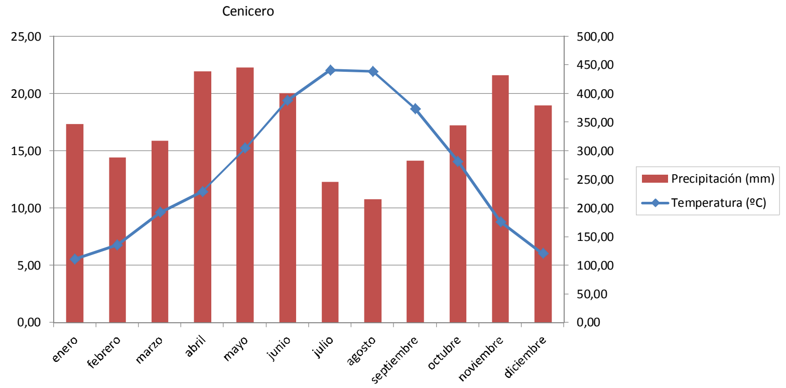
Gráfico 3 Diagrama ombrotérmico de Cenicero, 1975-2014
