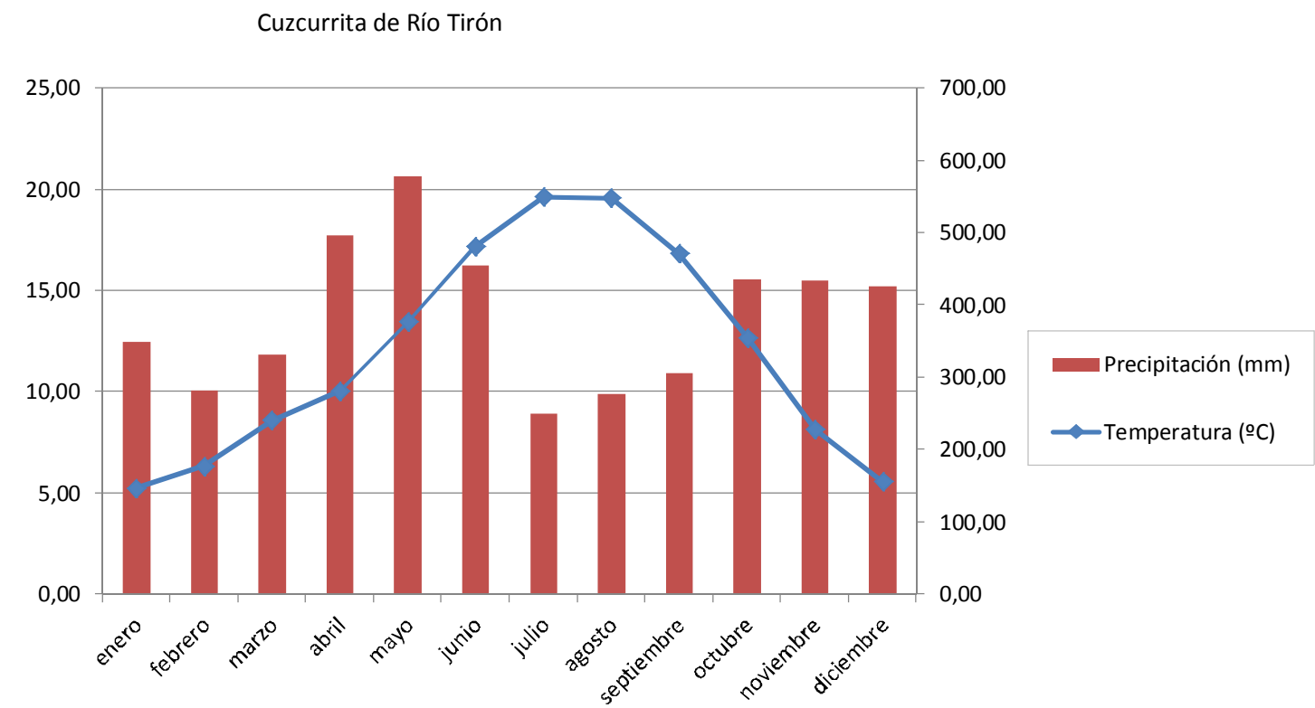
Gráfico 1 Diagrama ombrotérmico de Cuzcurrita de Río Tirón, 1975-2014
